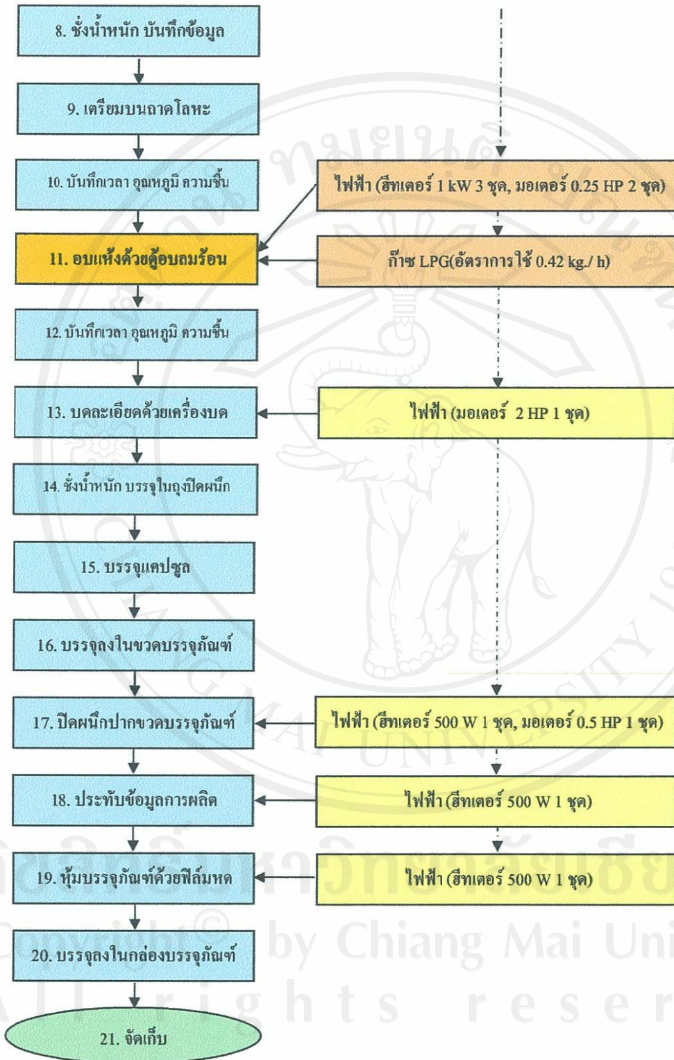
รูป 5.1 แผนภูมิแสดงขั้นตอนและกระบวนการผลิตสำหรับยาแก้ปวดและการใช้พลังงาน
