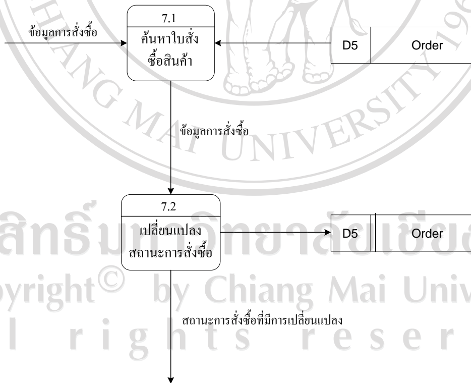
รูป 4.11 แผนผังกระแสข้อมูลระดับที่ 1 ของกระบวนการที่ 7 การเปลี่ยนแปลงสถานะการสั่งซื้อ
