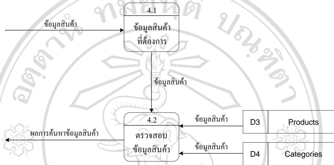
รูป 4.8 แผนผังกระแสข้อมูลระดับที่ 1 ของกระบวนการที่ 4การค้นหาข้อมูลสินค้า
