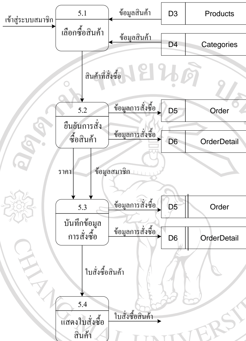
รูป 4.9 แผนผังกระแสข้อมูลระดับที่ 1 ของกระบวนการที่ 5 การสั่งซื้อสินค้า
