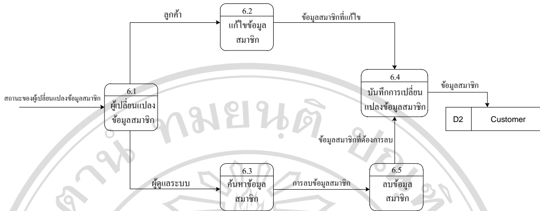
รูป 4.10 แผนผังกระแสข้อมูลระดับที่ 1 ของกระบวนการที่ 6 การแก้ไขข้อมูลสมาชิก (ลบ/แก้ไข)
