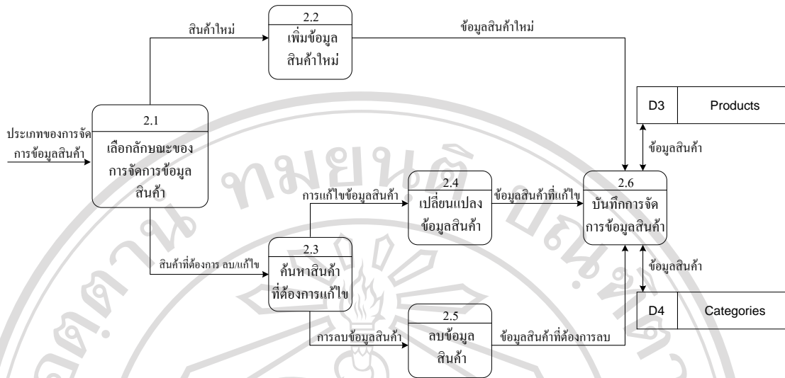
รูป 4.6 แผนผังกระแสข้อมูลระดับที่ 1 ของกระบวนการที่ 2 การจัดการข้อมูลสินค้า
