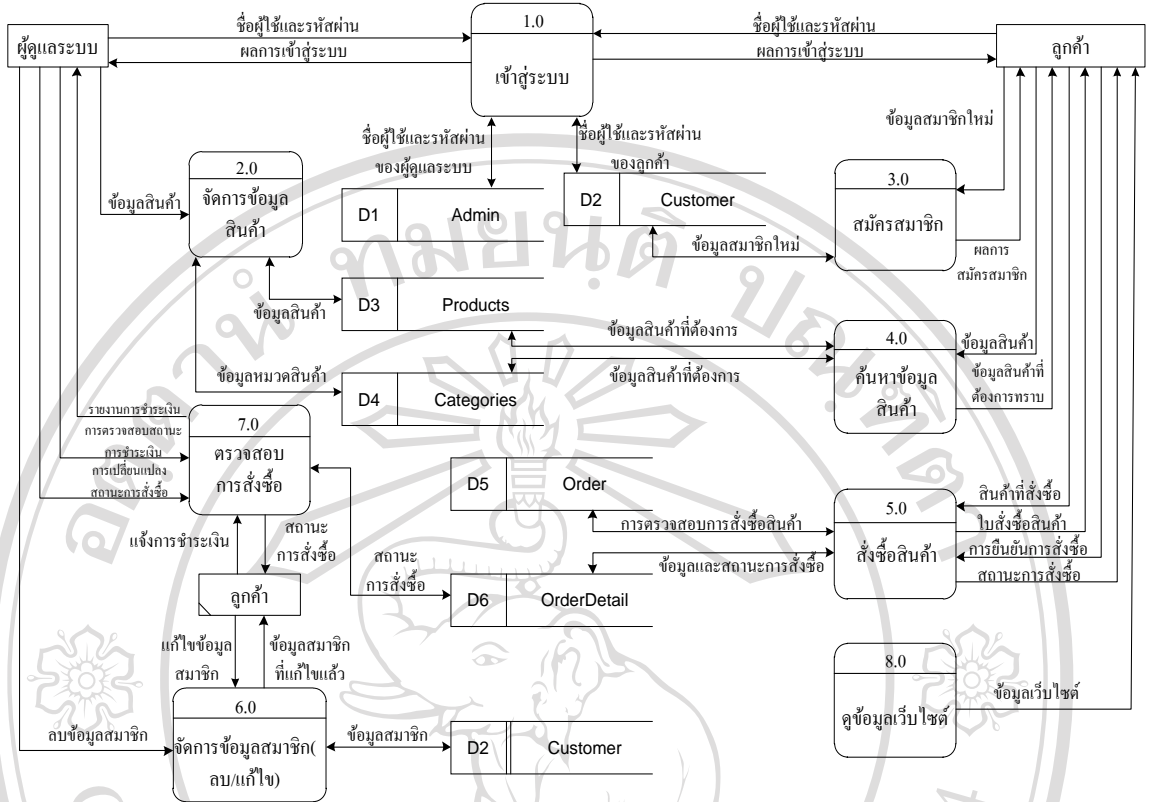
รูป 4.4 แผนผังกระแสข้อมูลระดับที่ 0 ระบบพาณิชย์อิเล็กทรอนิกส์บ้านหม้อแสนดีกราฟ
