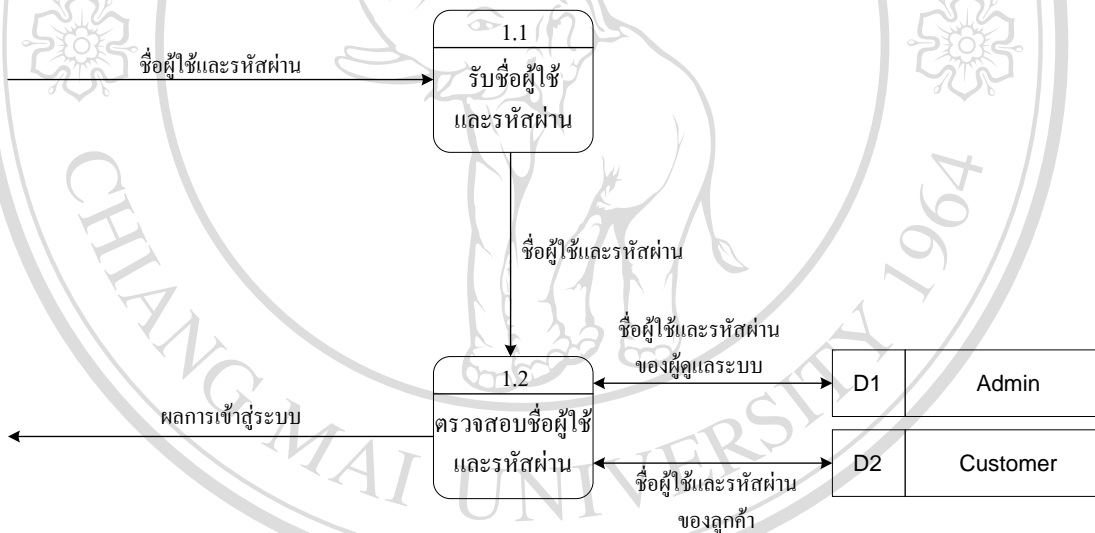
รูป 4.5 แผนผังกระแสข้อมูลระดับที่ 1 ของกระบวนการที่ 1 การเข้าสู่ระบบ
