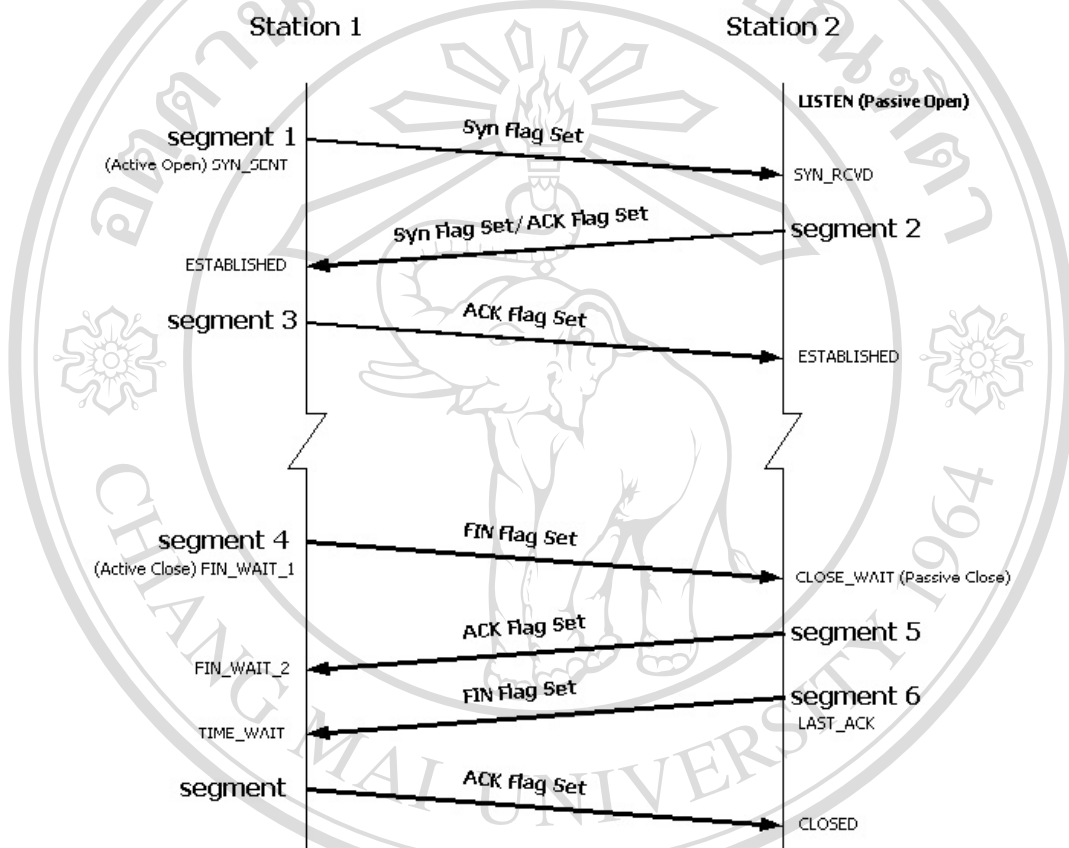
รูปที่ 2.8 แสดงลำดับและสถานะต่างๆของโปรโตคอล TCP ในการเริ่มต้นและสิ้นสุดการเชื่อมต่อ 5
