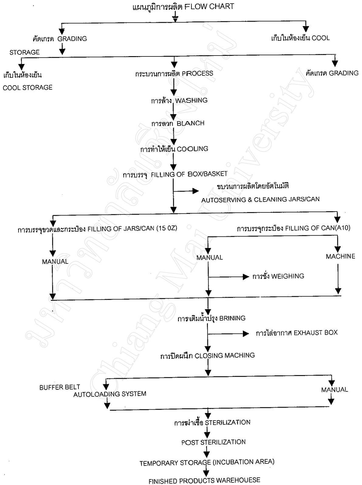
แผนภูมิที่ 3 : แสดงกระบวนการผลิตพริกผัก และผลไม้บรรจุภาชนะปิดผนึก
