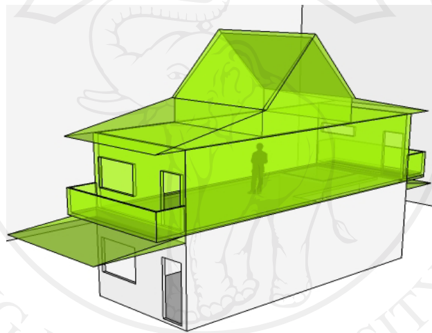
ภาพที่ 4.17 บ้านชั้นเดียวแบบต่อเป็นสองชั้นและกันสาดด้านหน้า
