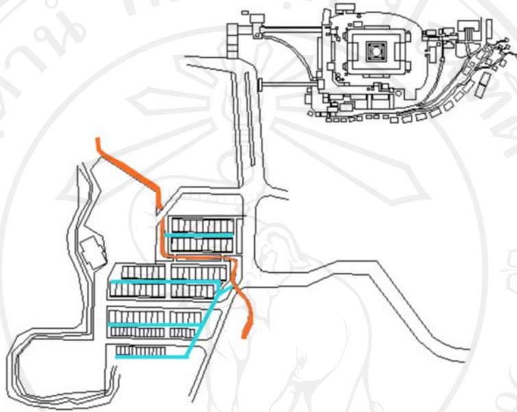
แผนผังที่ 4.6 แสดงเส้นทางระบายน้ำของชุมชน
