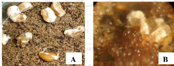
ภาพ 3-10 เชื้อรา B. bassiana ในข้าวฟ่างวันที่ 1 ของการทดลอง (A) และไข่เห็บ (B)
