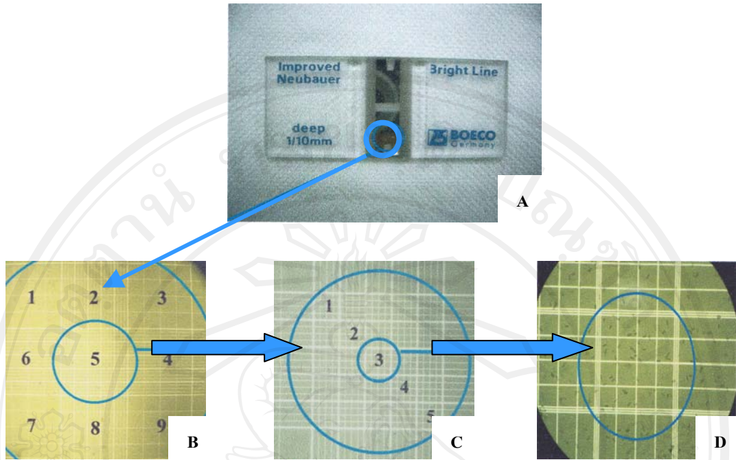
ภาพ 3-3 การนับสปอร์เชื้อราโดยใช้ Haemacytometer A คือ พื้นที่สำหรับการนับสปอร์เชื้อราอยู่ 2 chamber B คือ บริเวณที่ใช้สำหรับนับจะแบ่งออกเป็น 9 ช่อง C คือ การนับสปอร์เชื้อราในแต่ละchamber จะนับในแนวทแยงมุม D คือ ลักษณะของสปอร์เชื้อราที่ทำการนับ
