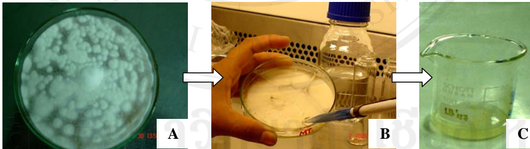
ภาพ 3-1 เชื้อรา B. bassiana ที่เลี้ยงไว้บนอาหาร MEA อายุ 14-21 วัน (A), การล้างสปอร์ (B) และสารแขวนลอยสปอร์ที่ผ่านการกรองด้วยผ้าขาวบาง (C)
