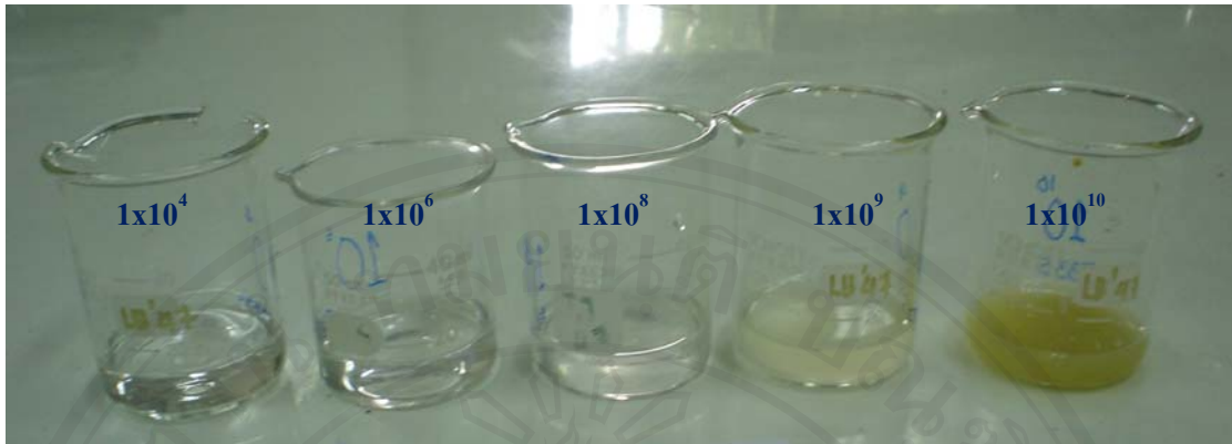
ภาพ 3-7 สารแขวนลอยสปอร์เชื้อรา B. bassiana ที่ระดับความเข้มข้น 1 \times 10^4 , 1 \times 10^6 , 1 \times 10^8 , 1 \times 10^9 และ 1 \times 10^{10} สปอร์ต่อมล. (เรียงจากซ้ายไปขวา)
