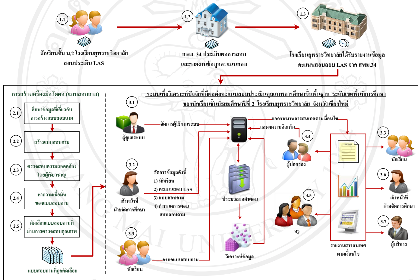
รูป 3.2 แสดงกระบวนการดำเนินการของระบบเพื่อวิเคราะห์คะแนนสอบประเมินคุณภาพการศึกษาขั้นพื้นฐาน ระดับเขตพื้นที่การศึกษา ของนักเรียนชั้นมัธยมศึกษาปีที่ 2 โรงเรียนยุพราชวิทยาลัย
