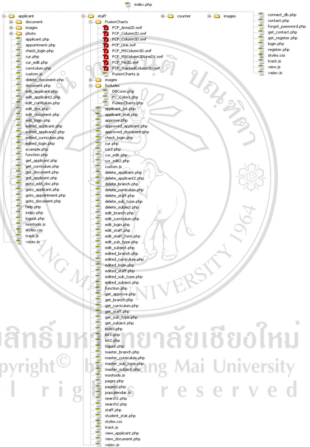
รูป 5.2 แผนผังโครงสร้างไฟล์โปรแกรม
