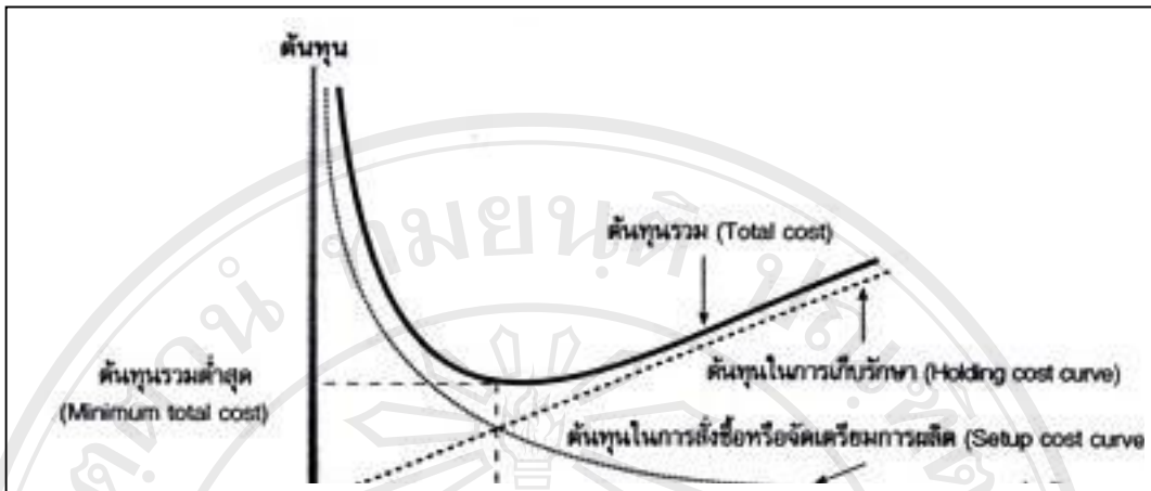
รูปที่ 2.3 แสดงความสัมพันธ์ระหว่างต้นทุนรวมกับปริมาณการสั่งซื้อ (Total cost as a function of quantity) (ประสงค์ ปรานีตพลกรังและคณะ,2544:261)
