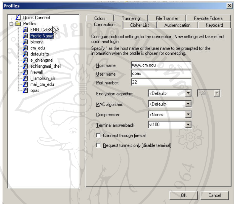
รูป ก.4 หน้าจอการติดตั้งค่าติดต่อกับเครื่องให้บริการเว็บ
