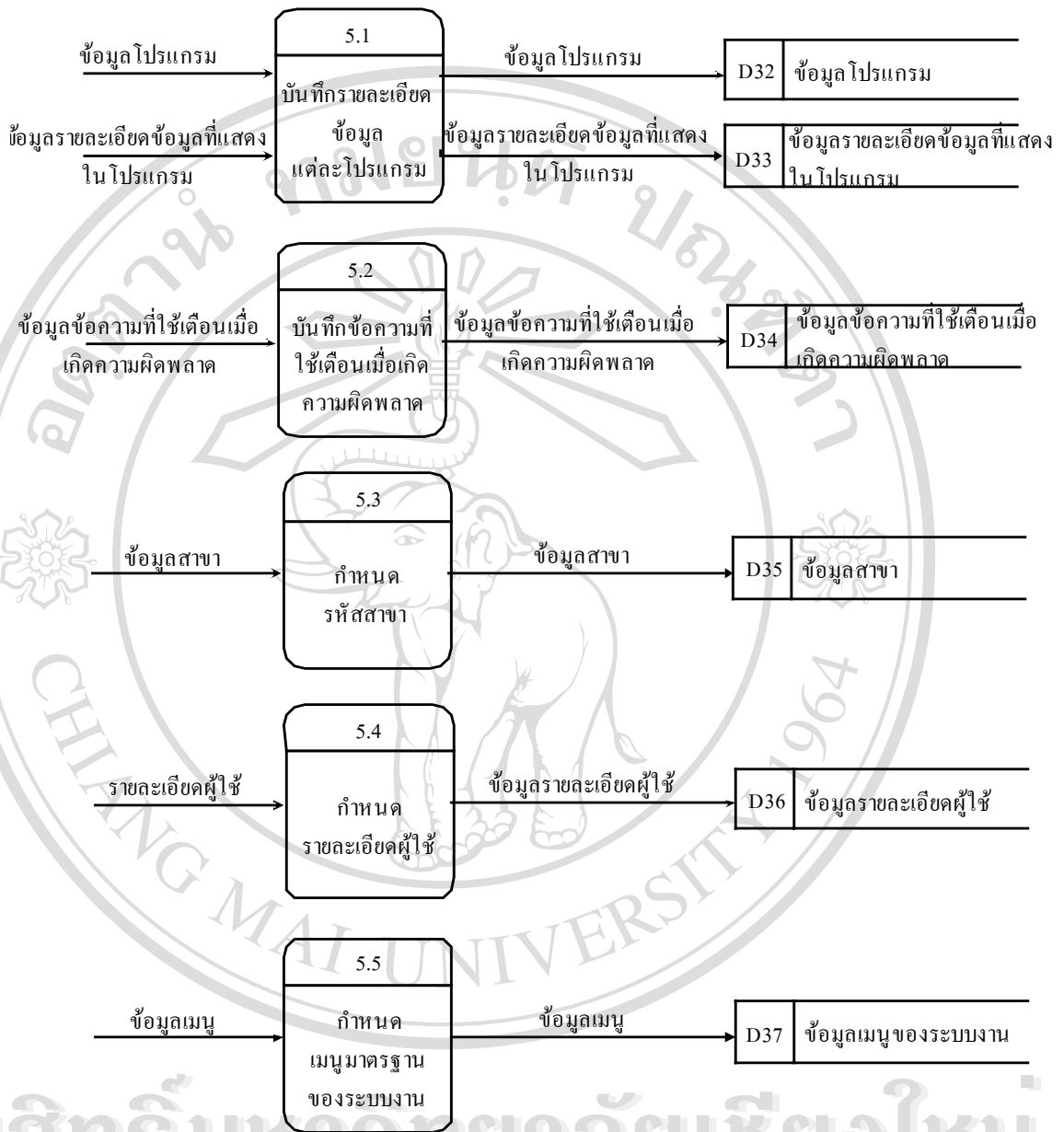
รูป 3.6 แสดงภาพดาต้าฟลั้วไดอะแกรมในระดับที่ 1 แสดงการบันทึกข้อมูลโปรแกรมระบบช่วยงาน
