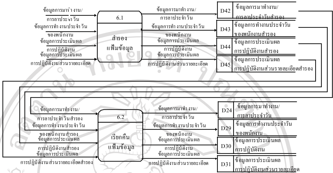
รูป 3.7 แสดงภาพดาต้าโฟลว์ไดอะแกรมในระดับที่ 1 แสดงการสำรองและเรียกคืนข้อมูล
