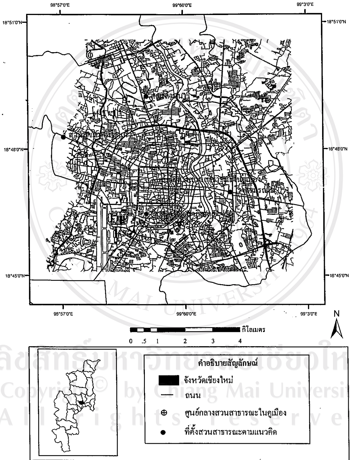
ภาพที่ 16 แสดงแนวคิิดการเพิ่มต้นไม้ในเมืองเขตเมืองเชียงใหม่
