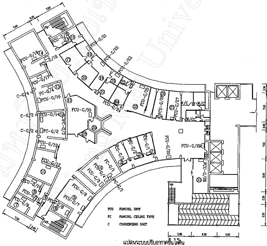
รูป 4.7 แสดงผังระบบปรับอากาศชั้นใต้ดิน
