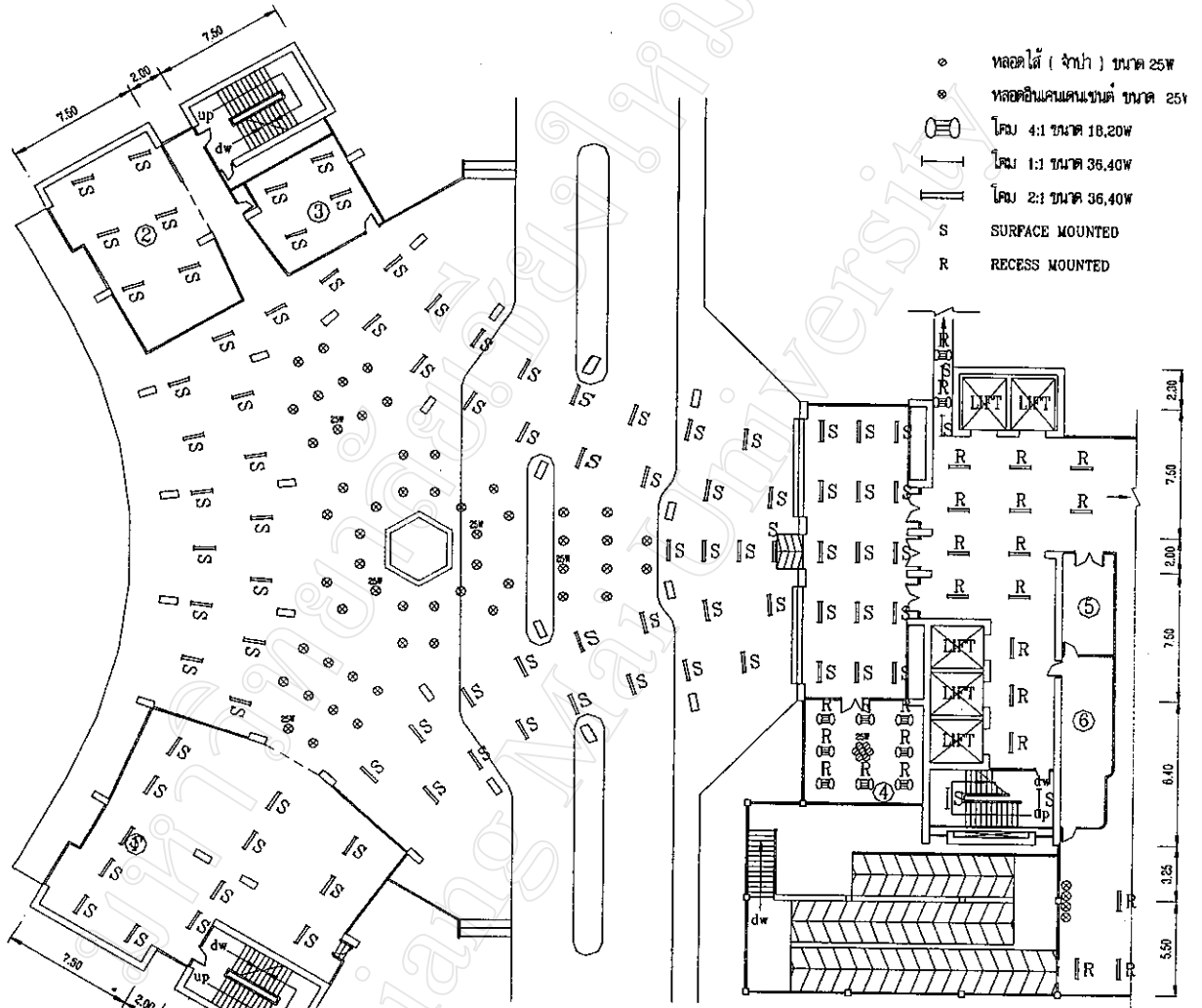
แปลนระบบไฟฟ้าชั้น 1
