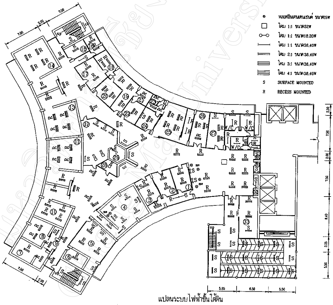
รูปภาคผนวก 3.1 แสดงผังระบบแสงสว่างชั้นใต้ดิน
