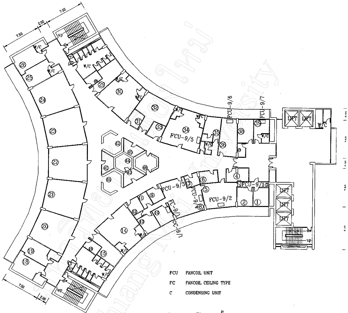
แปลนระบบปรับอากาศชั้น 9
