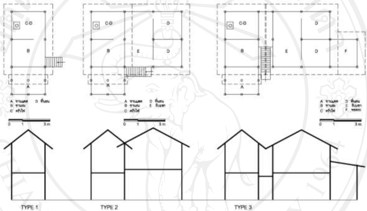
ภาพ 6-2 พัฒนาการของผังเรือนพักอาศัยของบ้านดง
