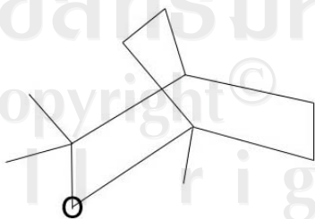
1,8-cineole
