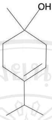
1-terpineol
