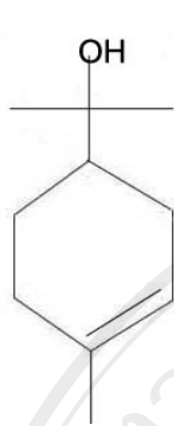
terpineol
