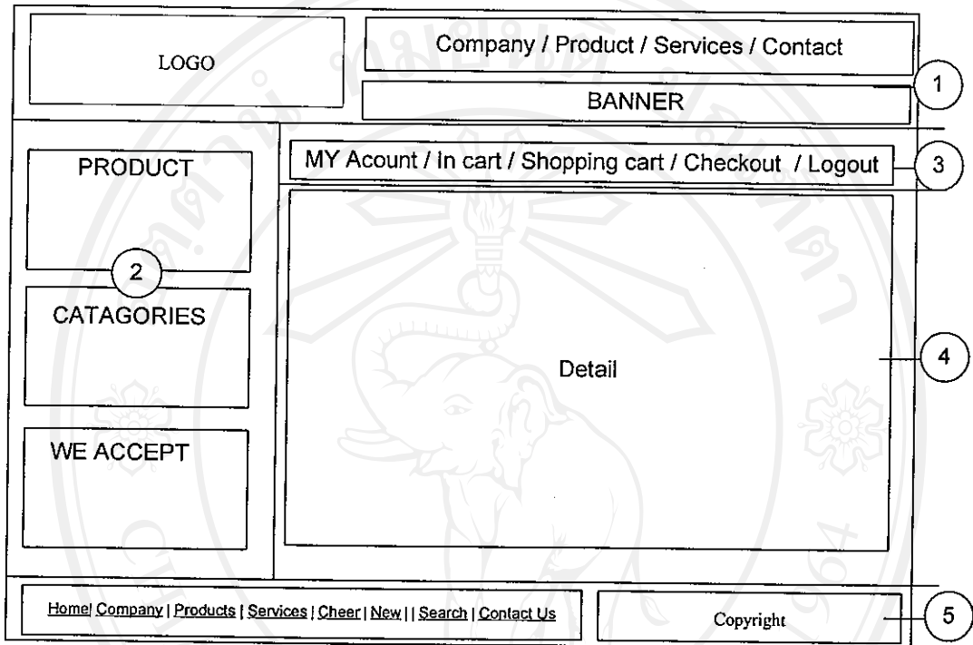
รูป 4.4 แสดงการออกแบบหน้าจอทั่วไปของส่วนหน้าร้าน
