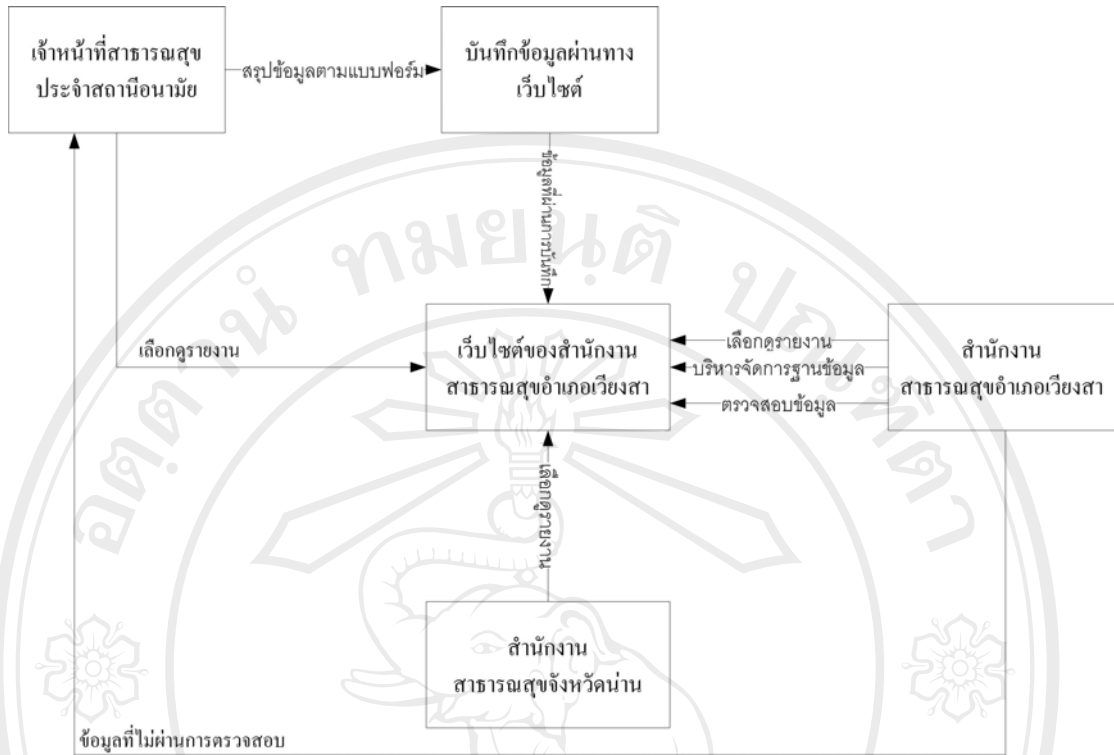
รูป 3.2 แสดงระบบจัดการข้อมูลในระบบงานใหม่
