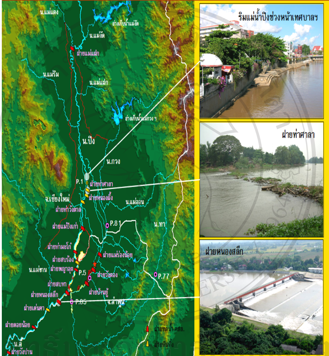
ภาพ 36 แสดงฝายต่างๆ จำนวน 12 ฝาย ที่กั้นลำน้ำแม่ปิง
