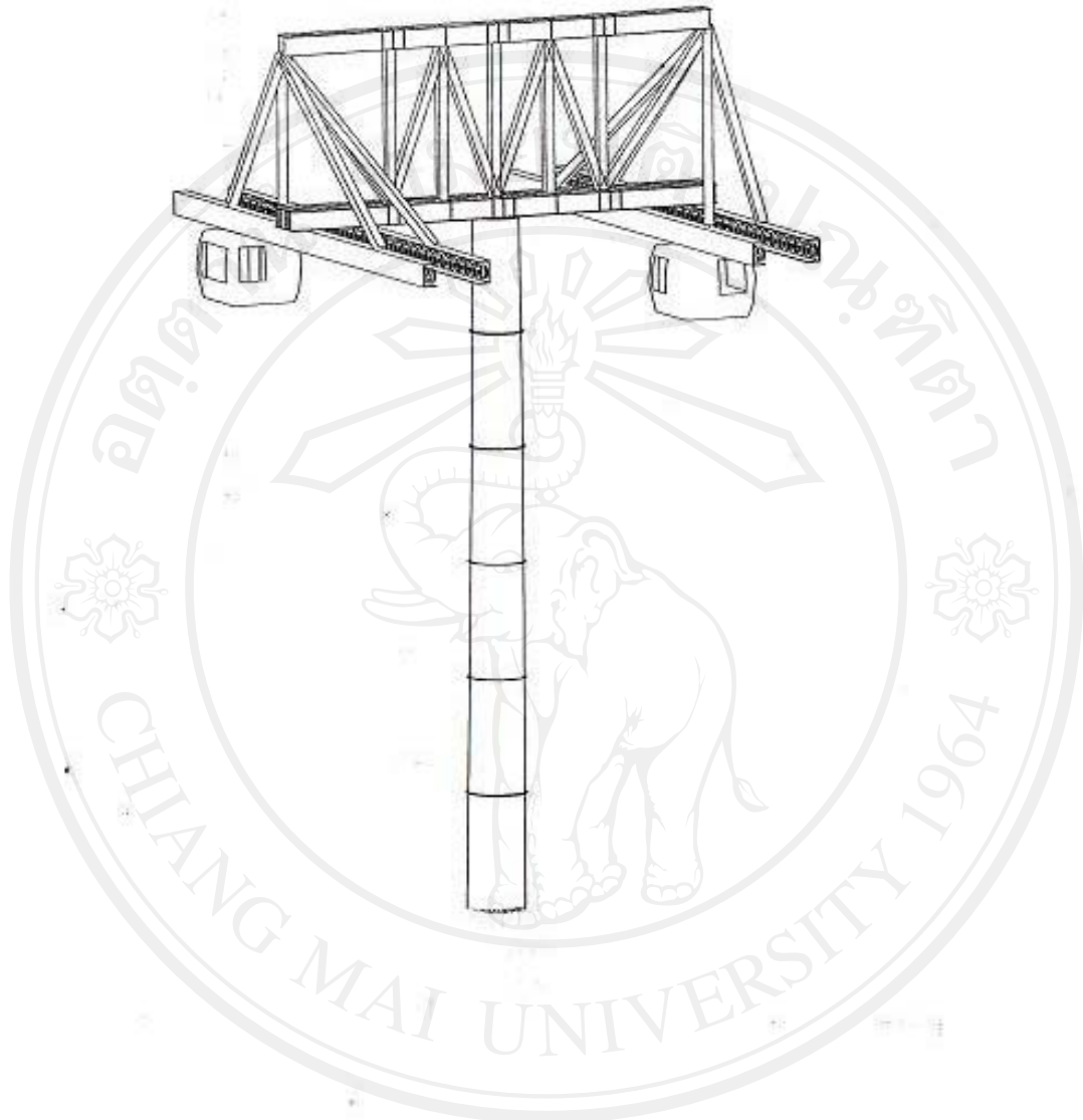
รูปภาพที่ 42 เสารับน้ำหนักแบบเสาเดี่ยวตั้งบนพื้นราบ ที่มา : บริษัท ปาย เคเบิ้ล ทรานสปอร์ต จำกัด, พฤศจิกายน 2550
