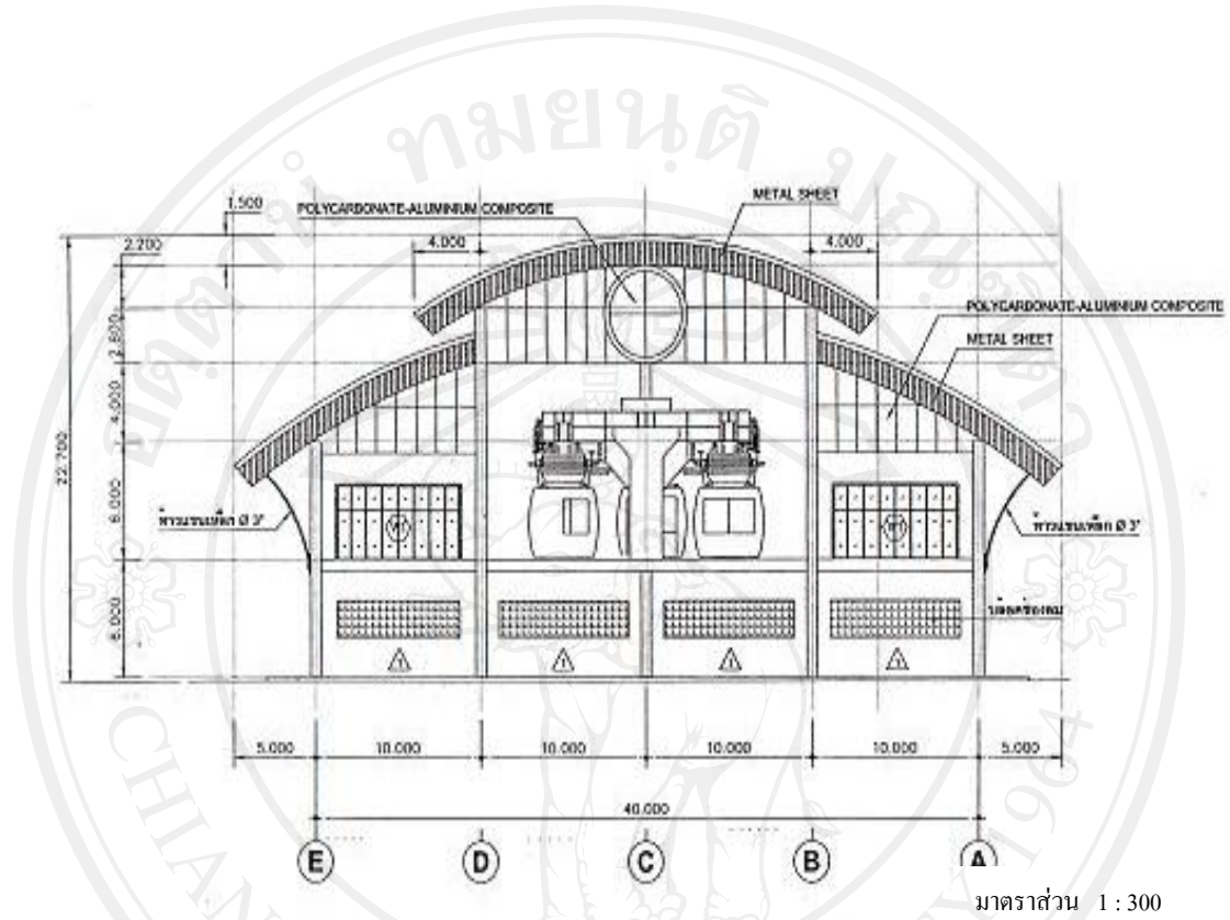
รูปภาพที่ 39 แบบแปลนรูปด้าน 1 สถานีระหว่างทาง ปาย ปางมะผ้า คอยก้างบอกไฟ ที่มา : บริษัท ปาย เคเบิ้ล ทรานสปอร์ต จำกัด, พฤศจิกายน 2
