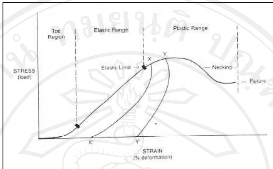
รูปที่ 1 แสดง stress-strain curve (Alter, 1990; นุชรีย์, 2542)
