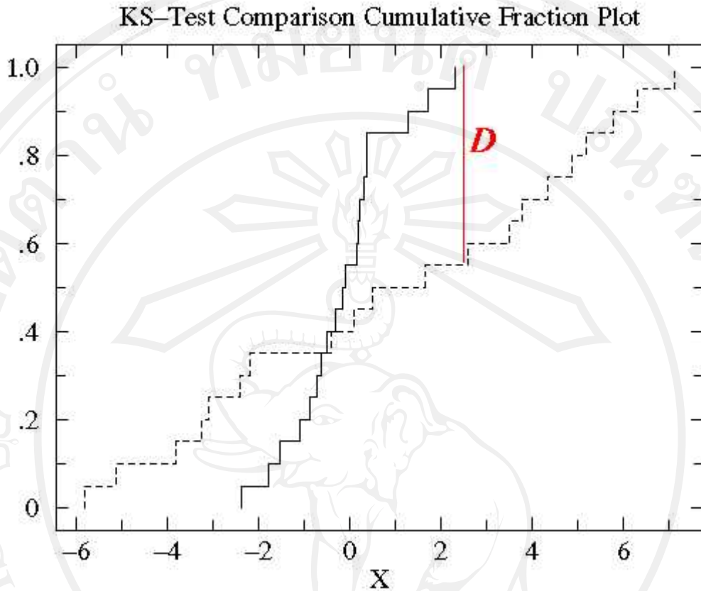
รูปที่ 3.1 แสดงตัวค่า D ระหว่างกราฟความถี่สะสมของข้อมูล 2 ชุด
