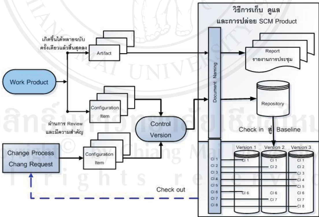
รูปที่ ก.2 แสดงตัวอย่างการบริหารจัดการการเปลี่ยนแปลงของข้อมูล
