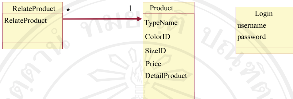
รูปที่ ก.18 แสดงคลาสไดอแกรมพร้อมแอททริบิวต์
