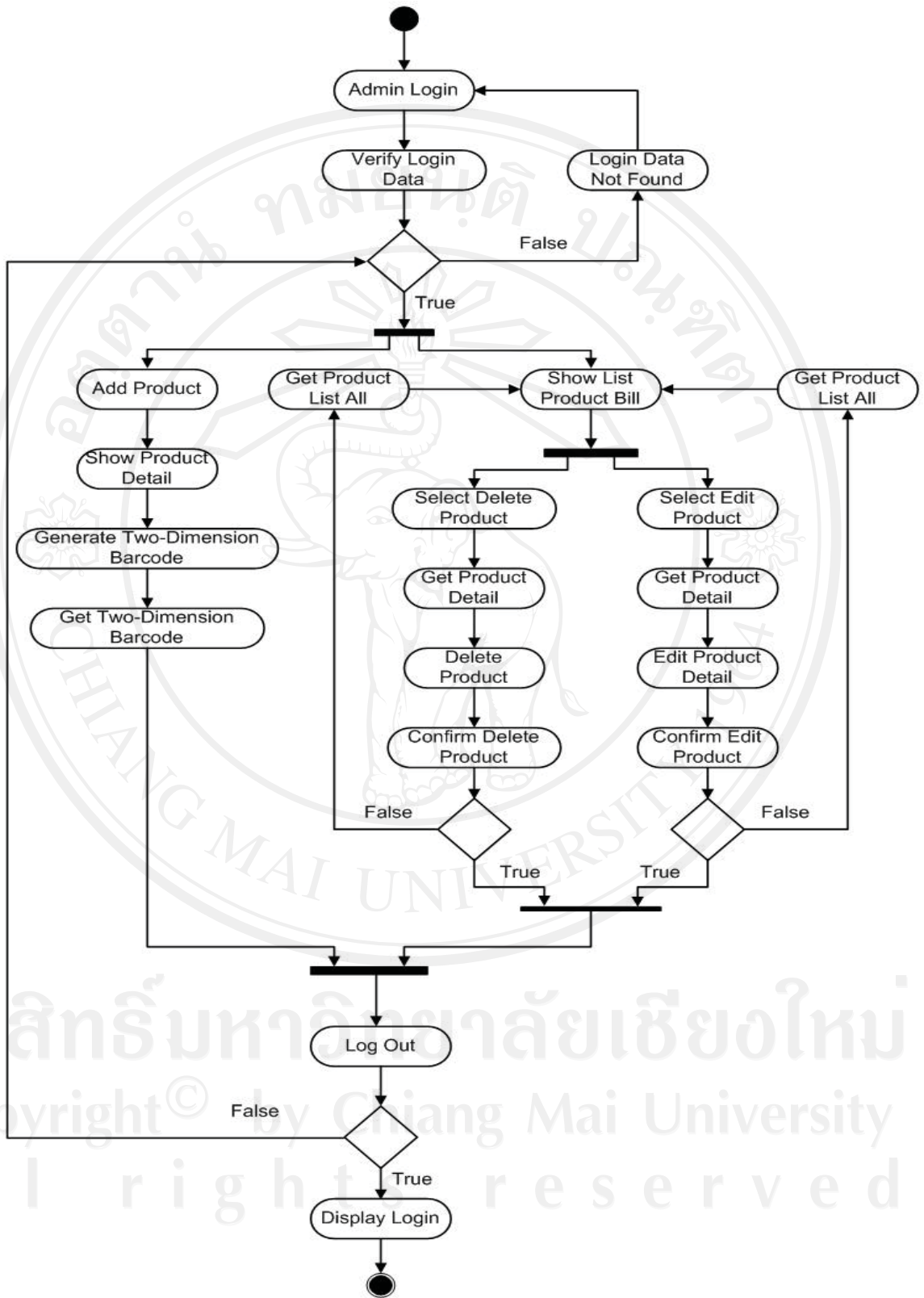
รูปที่ ก.20 แสดงแอกติวิตีไดอแกรมของผู้ดูแลระบบ
