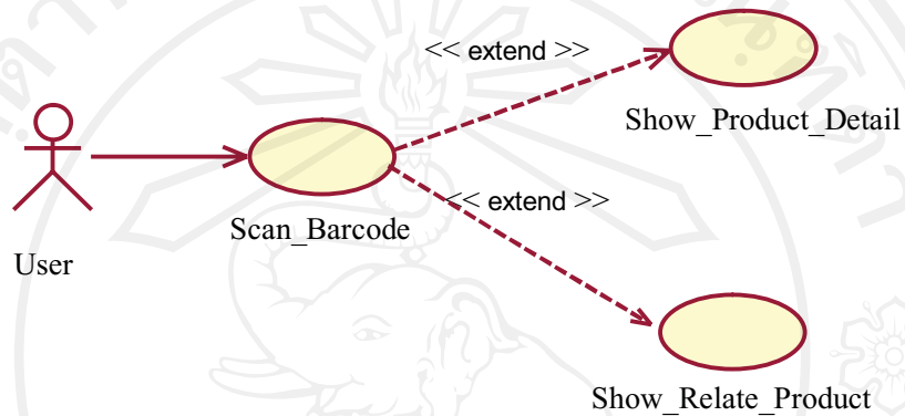
รูปที่ ก.8 แสดงการกำหนดความสัมพันธ์ของยูสเคส Scan_Barcode , Show_Product_Detail และ Show_Relate_Product
