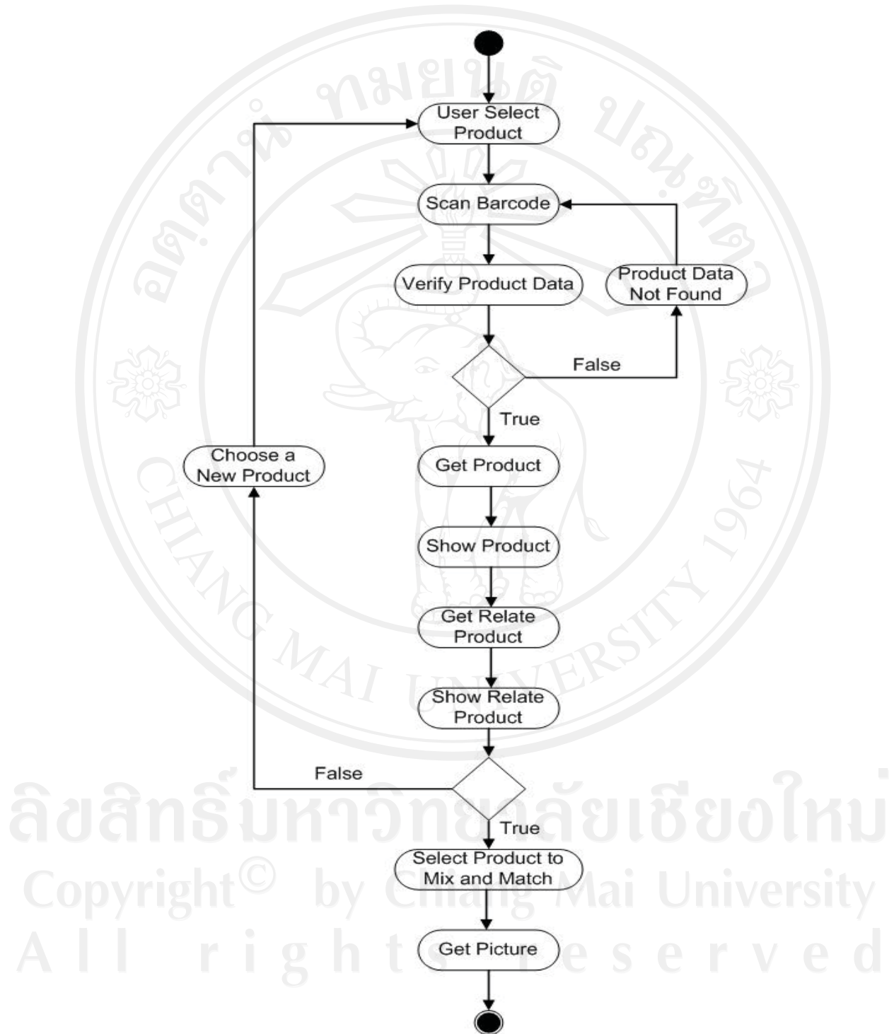
รูปที่ ก.19 แสดงเอกวิทัศน์ไดอแกรมของผู้ใช้งานทั่วไป
