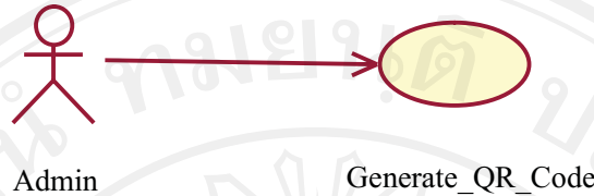
รูปที่ ก.13 แสดงการกำหนดความสัมพันธ์ของยูสเคส Generate_QR_Code
