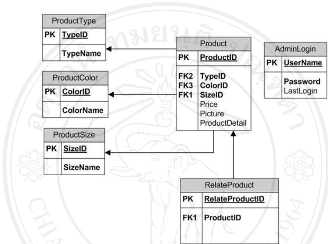
รูปที่ ก.21 แสดง อีอาร์ไดอะแกรม(ER – Diagram) ของระบบช่วยตัดสินใจสำหรับการเลือกเสื้อผ้าเครื่องแต่งกาย โดยใช้บาร์โค้ดสองมิติ
