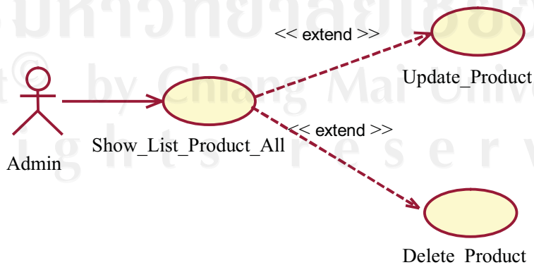
รูปที่ ก.12 แสดงการกำหนดความสัมพันธ์ของยูสเคส Show_List_Product_All , Update_Product และ Delete_Product
