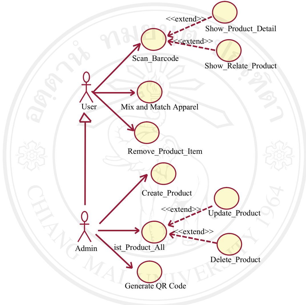
รูปที่ ก.4 แสดงการทำงานของยูสเคสระบบช่วยตัดสินใจสำหรับการเลือกเสื้อผ้าเครื่องแต่งกาย ลิขสิทธิ์มหาวิทยาลัยเชียงใหม่ โดยใช้บาร์โค้ดสองมิติ Copyright© by Chiang Mai University All rights reserved
