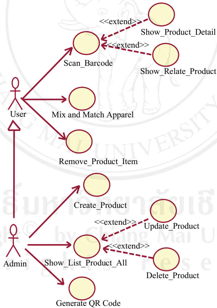
รูปที่ ก.15 แสดงการทำงานของยูสเคสระบบช่วยตัดสินใจสำหรับการเลือกเสื้อผ้าเครื่องแต่งกายโดยใช้บาร์โค้ดสองมิติ
