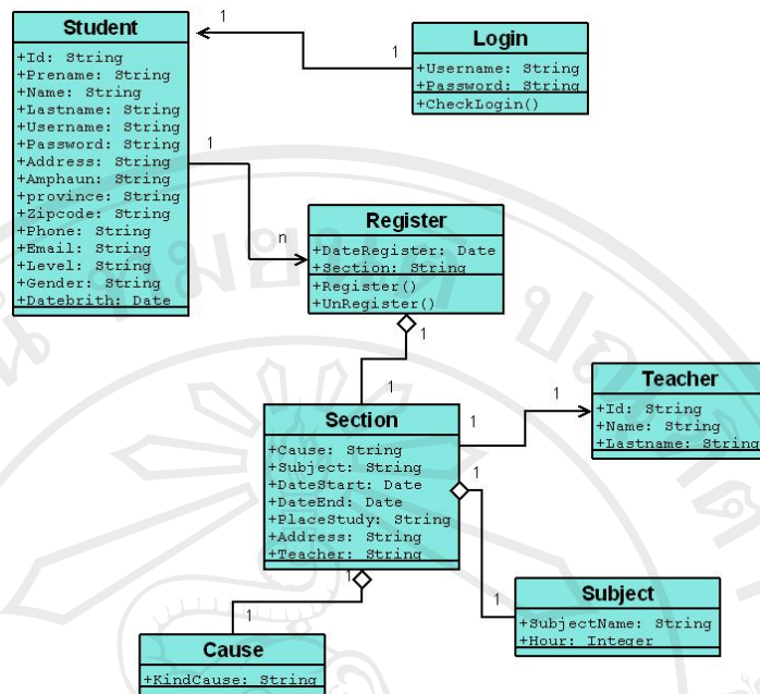
รูปที่ 5.1 คลาสไดแกรมของระบบลงทะเบียนออนไลน์
