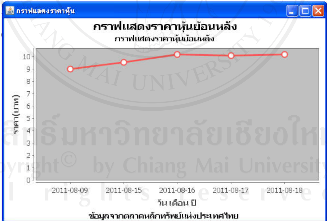
รูป ข.31 ตัวอย่างกราฟแสดงผลลัพธ์
