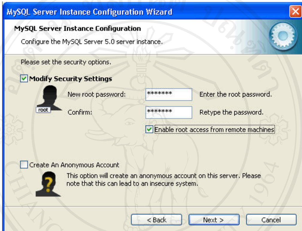
รูป ก.12 กำหนดรหัสผ่าน
